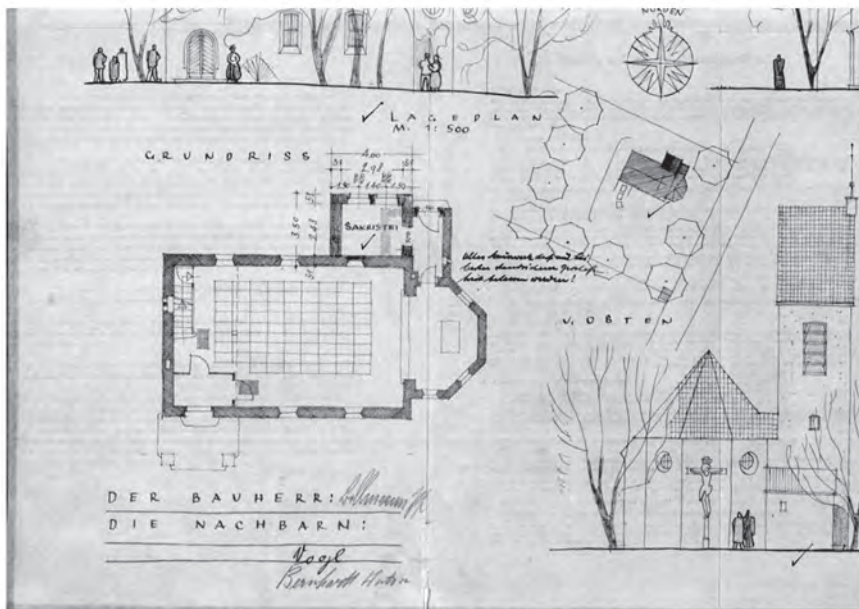
Ausschnitte des Plans von Regierungsbaumeister R. Dorn aus Regensburg vom Februar 1951 (Repro: Michaela Zeitler)
