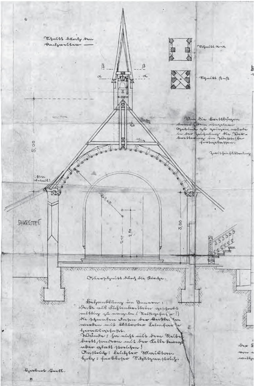
Entwurf von Herbert Prell vom 19.4.1939 (Repro: Michaela Zeitler)
