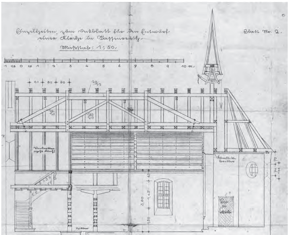
„Einzelheiten zum Deckblatt für den Entwurf einer Kirche in Sassenreuth“ von Herbert Prell vom 19.4.1939 (Repro: Michaela Zeitler)
